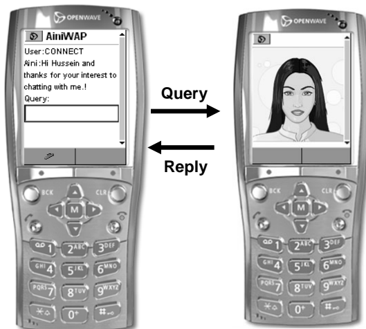
Fig. 13 WAPChat Interface
