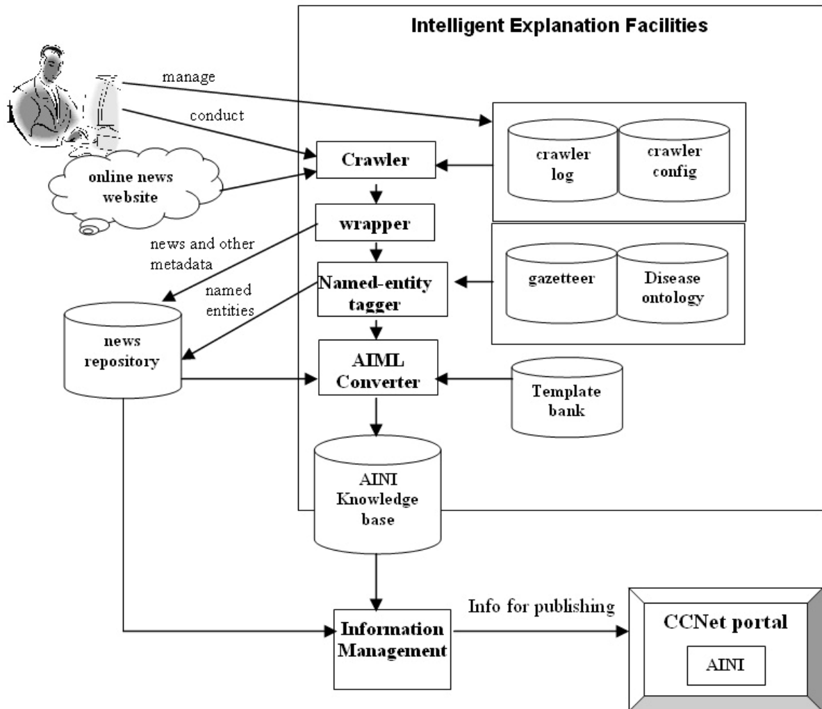
Fig. 3 AKEA Framework
