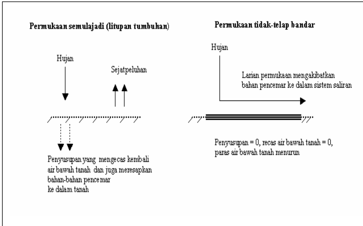
Rajah 1: Perbezaan konseptual perubahan hidrologi di antara permukaan semulajadi dan tepubina bandar (Sumber: Noorazuan & Siti Aisah, 2006).
