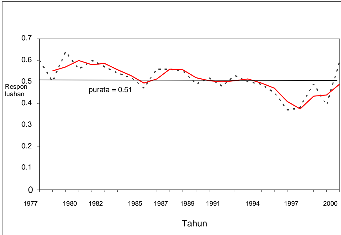
Rajah 11: Variasi tahunan respon luahan. Garis merah merujuk kepada nilai 3-tahun purata bergerak.
