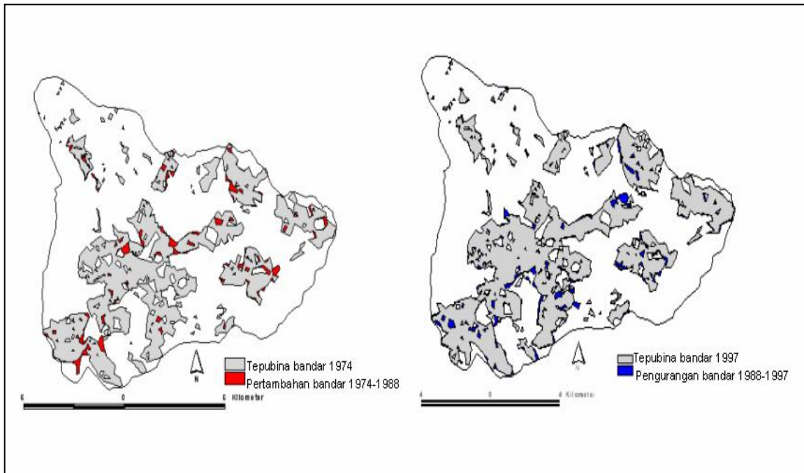
Rajah 10: Pertambahan kawasan tepubina akibat rebakan bandar (1974-1988) dan pengurangan kawasan tepubina akibat fasa rejuvenasi bandar (1988-1997) dalam Lembangan Sankey (Noorazuan, 2006).
