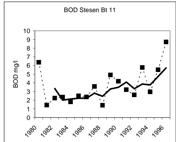
Rajah 4: Perubahan kepekatan BOD yang dicerap di kedua-dua sub-lembangan di antara 1980 hingga 1996. Nota: Garis hitam merujuk kepada nilai 3-tahun purata bergerak BOD.
