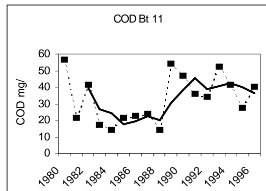
Rajah 5: Perubahan kepekatan COD dalam kedua-dua sub-lembangan di antara 1980 hingga 1996. Nota: Garis hitam merujuk kepada nilai 3-tahun purata bergerak COD.
