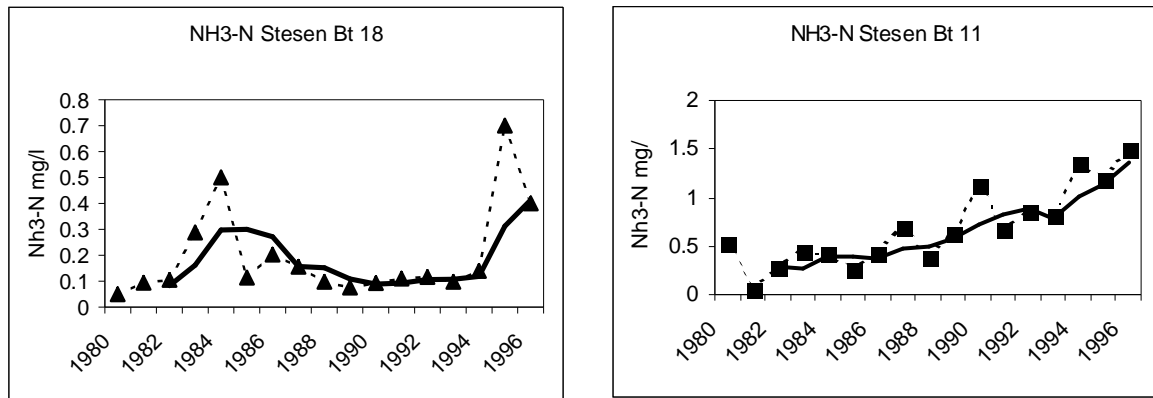
Rajah 6: Perubahan kepekatan Ammonikal-Nitrogen (AN) dalam kedua-dua sub-lembangan diantara 1980 hingga 1996. Nota: Garis hitam merujuk kepada nilai 3-tahun purata bergerak AN.
