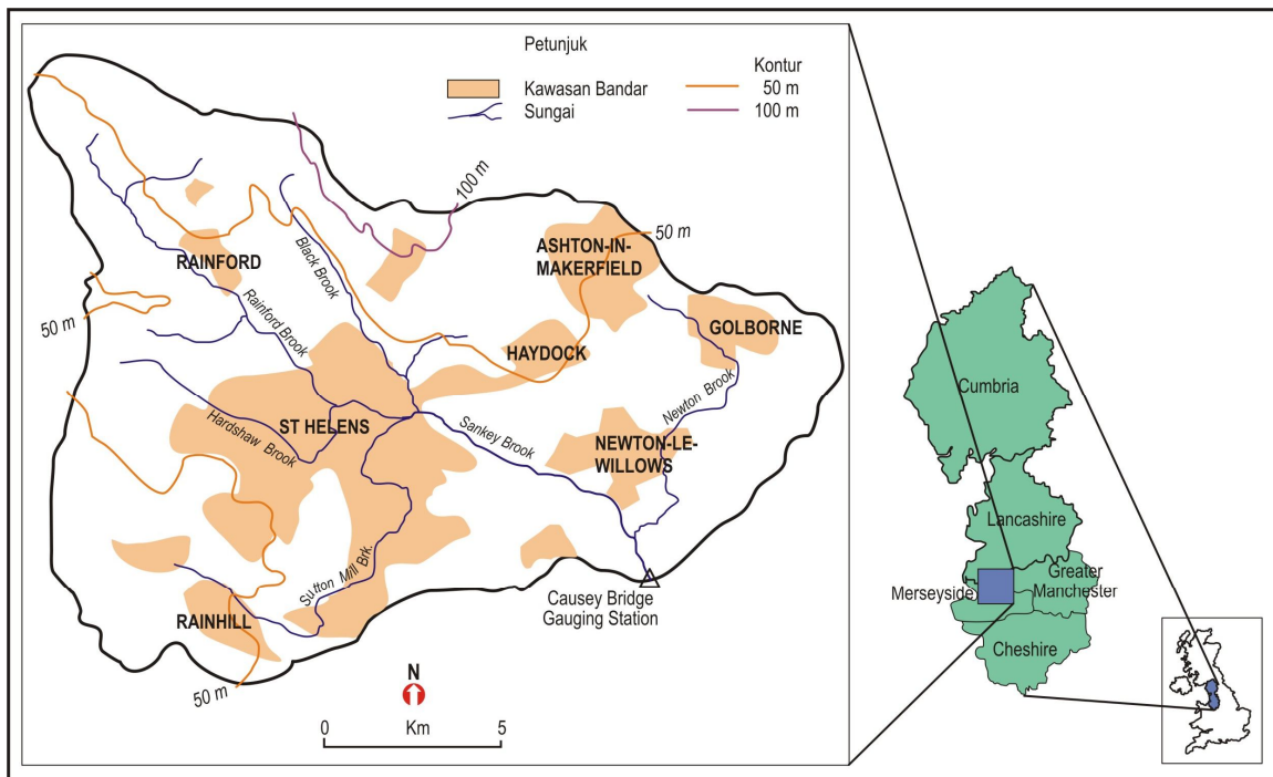
Rajah 3: Letakan bandar-bandar utama dalam Lembangan Sg Sankey (Noorazuan 2006)
