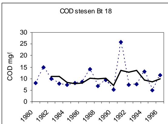
Rajah 5: Perubahan kepekatan COD dalam kedua-dua sub-lembangan di antara 1980 hingga 1996. Nota: Garis hitam merujuk kepada nilai 3-tahun purata bergerak COD.
