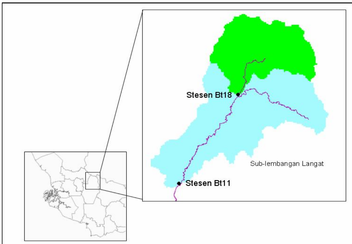
Rajah 2: Kawasan kajian di sub-lembangan Langat, i) kawasan tadahan stesen Bt 11 dan ii) kawasan tadahan Stesen Bt 18. Sumber: Noorazuan (1998)
