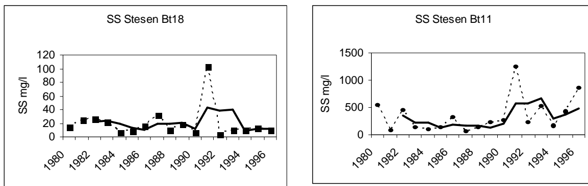
Rajah 7: Perubahan kepekatan pepejal terampai (SS) dalam kedua-dua sub-lembangan diantara 1980 hingga 1996. Nota: Garis hitam merujuk kepada nilai 3-tahun purata bergerak SS.
