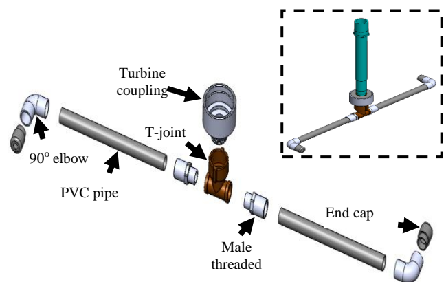
Fig. 1. Z-Blade turbine
