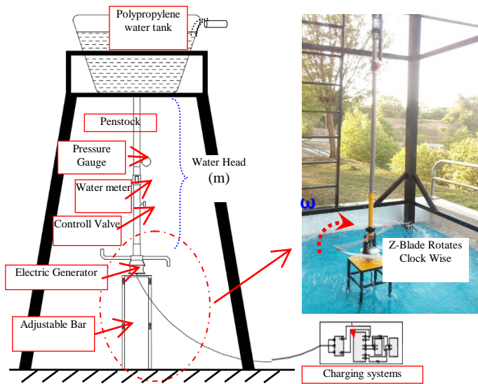
Fig. 3. Z-Blade turbine test rig
