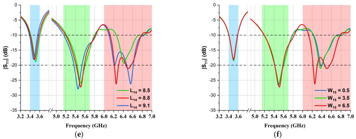
Figure 3. Parametric analysis of the presented MIMO multiband antenna. (a) W_8 ; (b) W_{11} ; (c) L_7 ; (d) L_4 ; (e) L_{14} ; (f) W_{15} .
