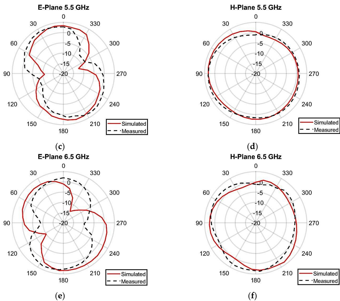
Figure 12. Radiation pattern of presented MIMO multiband antenna: (a) E-plane (3.50 GHz), (b) H-plane (3.50 GHz), (c) E-plane (5.50 GHz), (d) H-plane (5.50 GHz), (e) E-plane (6.50 GHz), (f) H-plane (6.50 GHz).
