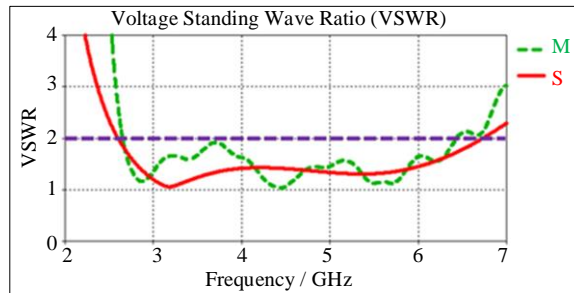
(d) VSWR
