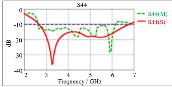
(f) A4
