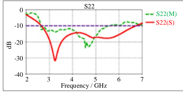
(d) A2
