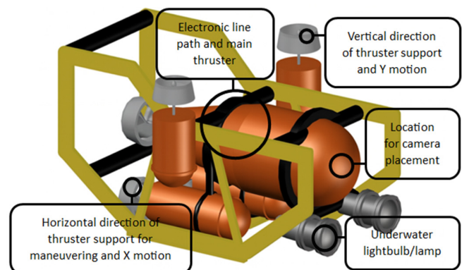
Fig. 1. ROV profile.
