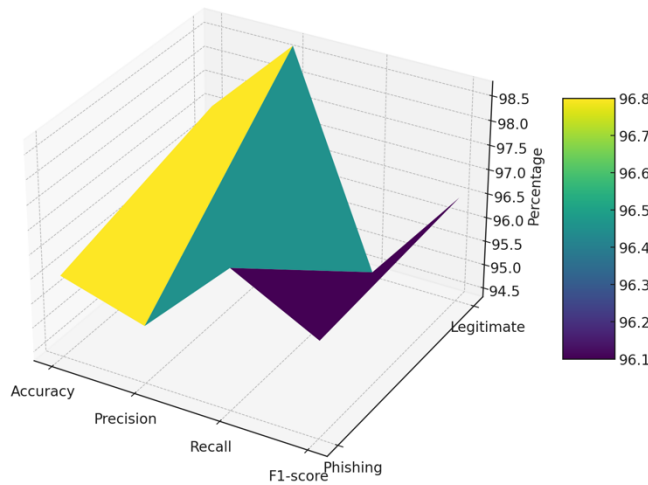
Fig. 4. Evaluation Metrics
