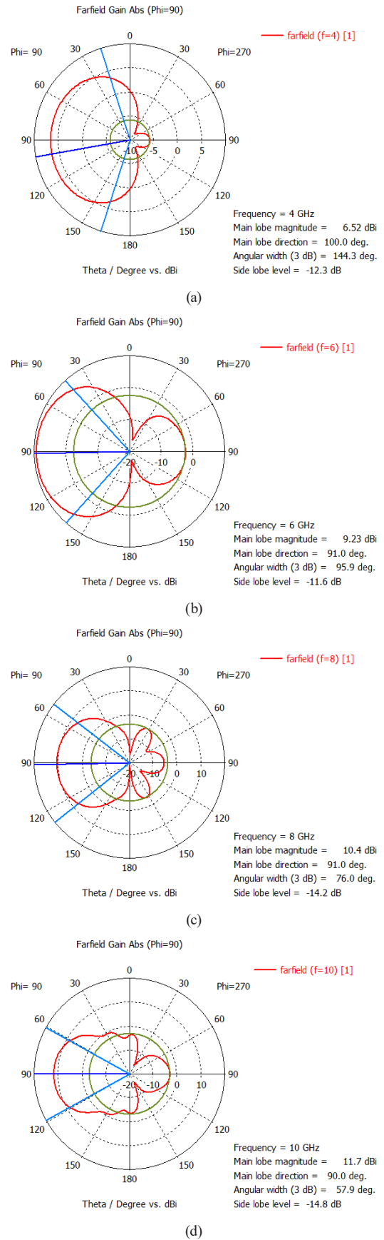
Fig. 2 Far-field directivity plots of SAVA, (a) 4 GHz, (b) 6 GHz, (c) 8 GHz, (d) 10 GHz
